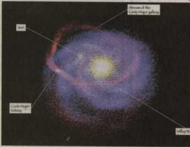
ดาวจักรแคระหมู่ใหญ่(ซีธรมู) กำลังถูกดาวจักรทางช้างเผือกคยยี่เป็นเสียง จากการจำลองด้วยคอมพิวเตอร์พบว่า ภายในเวลา 2,000 ล้านปี ดาวของดาวจักรแคระจะหลุดออกมาเป็นสายพันรอบดาวจักรทางช้างเผือก(สีฟ้า) ได้สามรอบ (ภาพจาก Nicolas Martin & Rodrigo Ibata/Strasbourg Observatory
