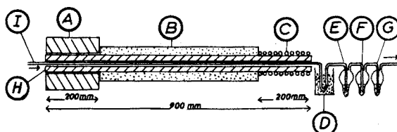
Fig. 1. A, four électrique; B, calorifuge; C, serpentin de refroidissement; D, piège à glace + NaCl; E et F, flacons laveur à HCl conc.; G, flacon laveur à \text{HNO}_3 conc.; H, tube de cuivre; I, tube de quartz.
