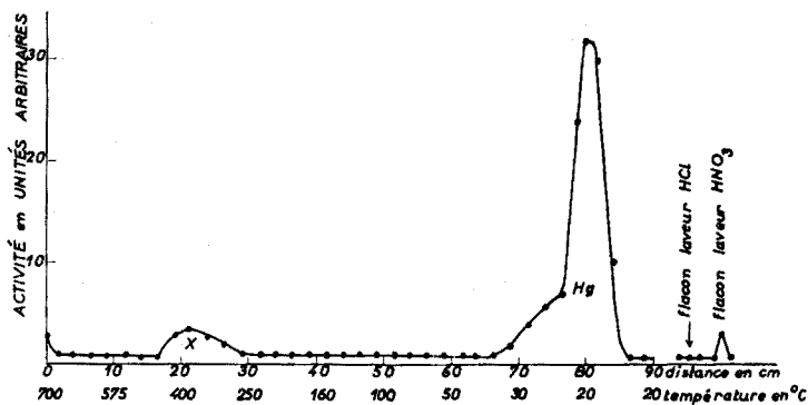
Fig. 4. Séparation de Hg (atmosphère d'argon, température du four: 700°).
