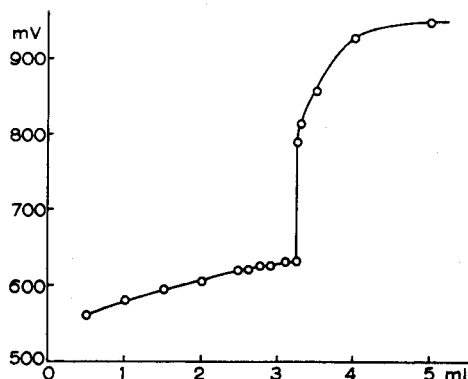
Fig. 2a Titration de 15 mg d'acide urique par le periodate de potassium dans un milieu de HCl à 15%.
