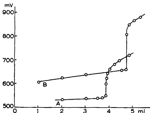
Fig. 1. Titrage de 15 mg d'acide urique par l'iodate de potassium, (A) dans un milieu de HCl à 0.8% (réduction en \text{I}_2 ), (B) dans un milieu de HCl à 15% (réduction en \text{ICl} ).
