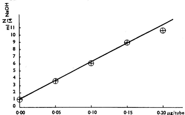
Fig. 1. Riboflavin
