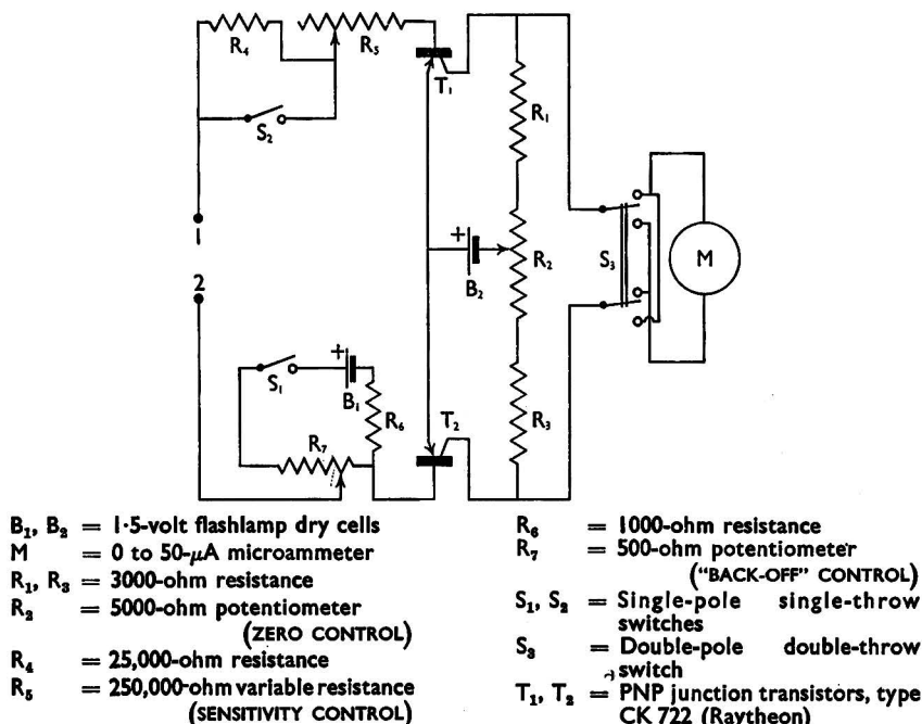
Fig. 1. Circuit diagram of titrimeter
